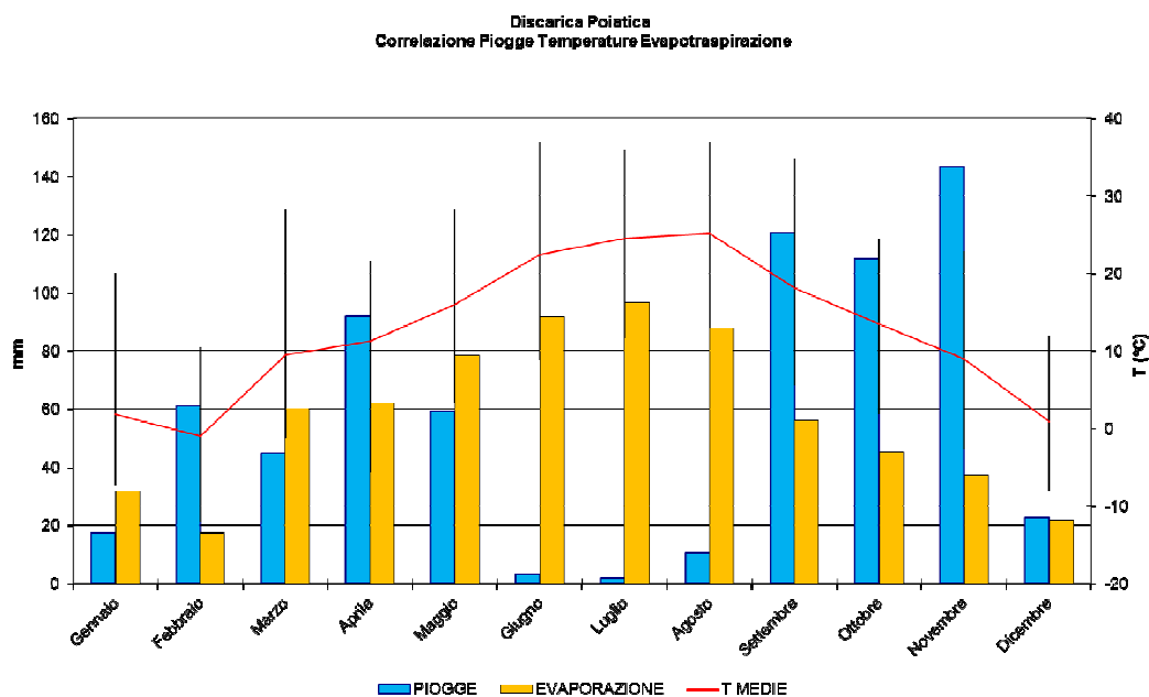
Grafico. n. 7 – Andamento di Temperatura, Evapotraspirazione e piovosità rilevati presso la Discarica di Poiatica, anno 2012
