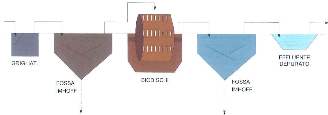
SCHEMA RETICOLO FOGNARIO
