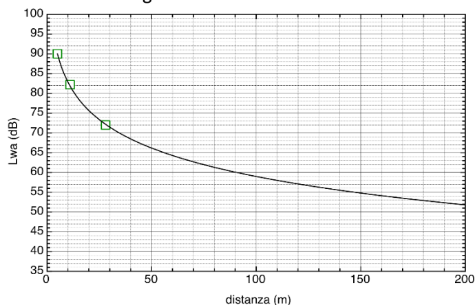
Figura 4.1 Curva di attenuazione per il livello di vibrazione stimata per una sorgente con L_{a,w} = 90 dB, nel range di distanza 0-200 m.
