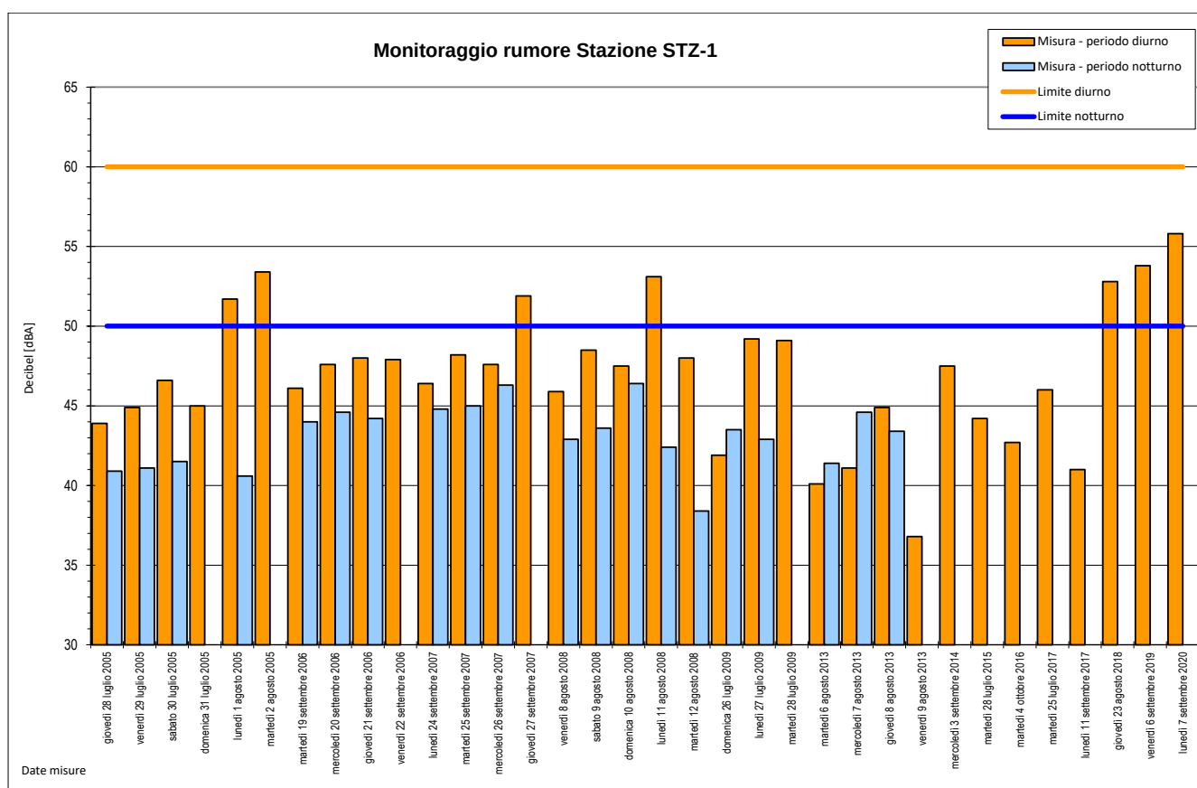
Figura 2.6. Estratto risultati monitoraggio acustico presso stazione STZ1 – Anni 2005-2020
