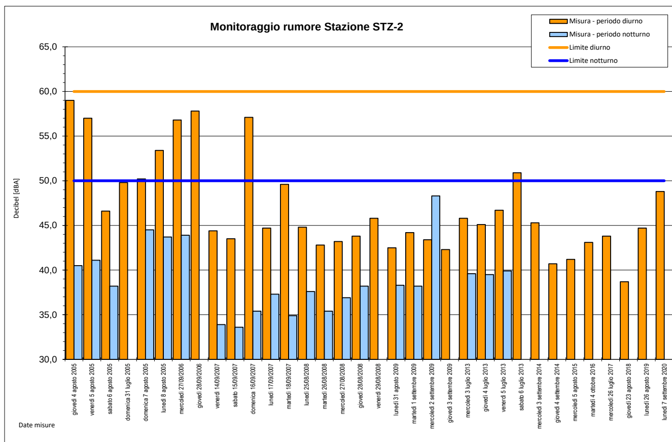
Figura 2.7. Estratto risultati monitoraggio acustico presso stazione STZ2 – Anni 2005-2020
