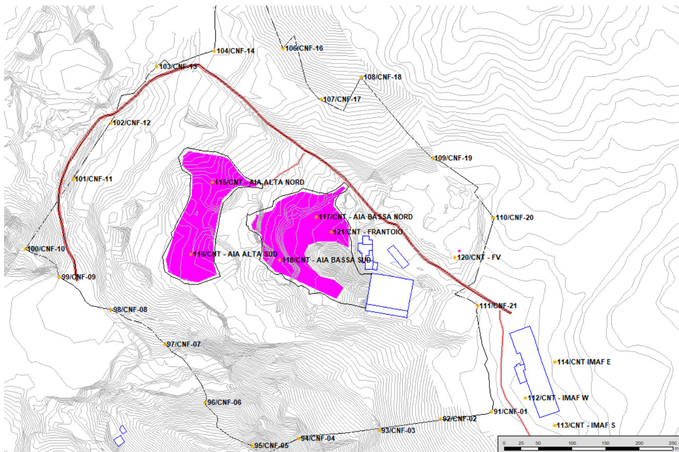
Figura 3.1. Estratto dal modello di simulazione acustica relativa alle aree di cava
