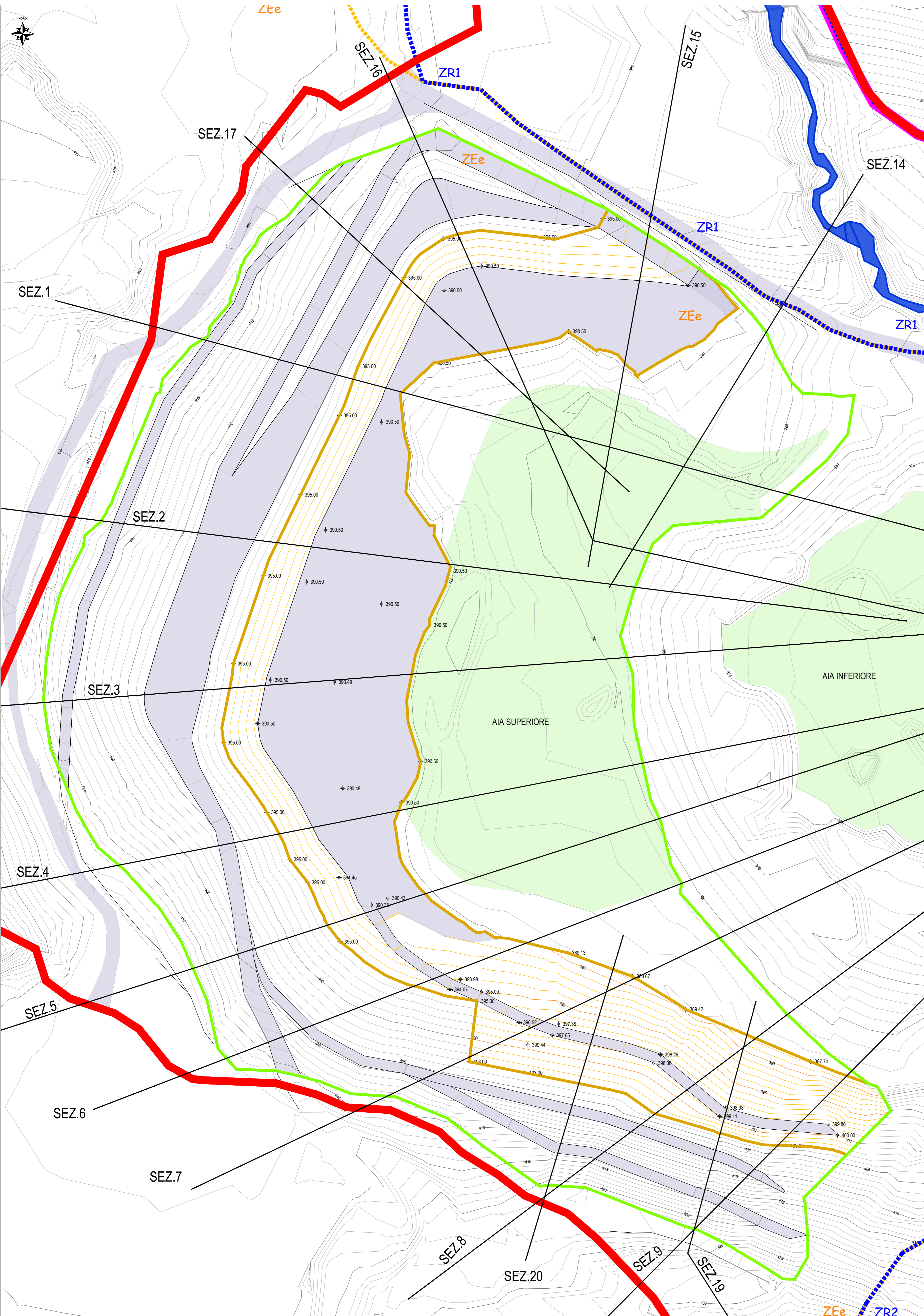
PLANIMETRIA DI PROGETTO DI COLTIVAZIONE - ANNO 3 - SCALA 1:750
