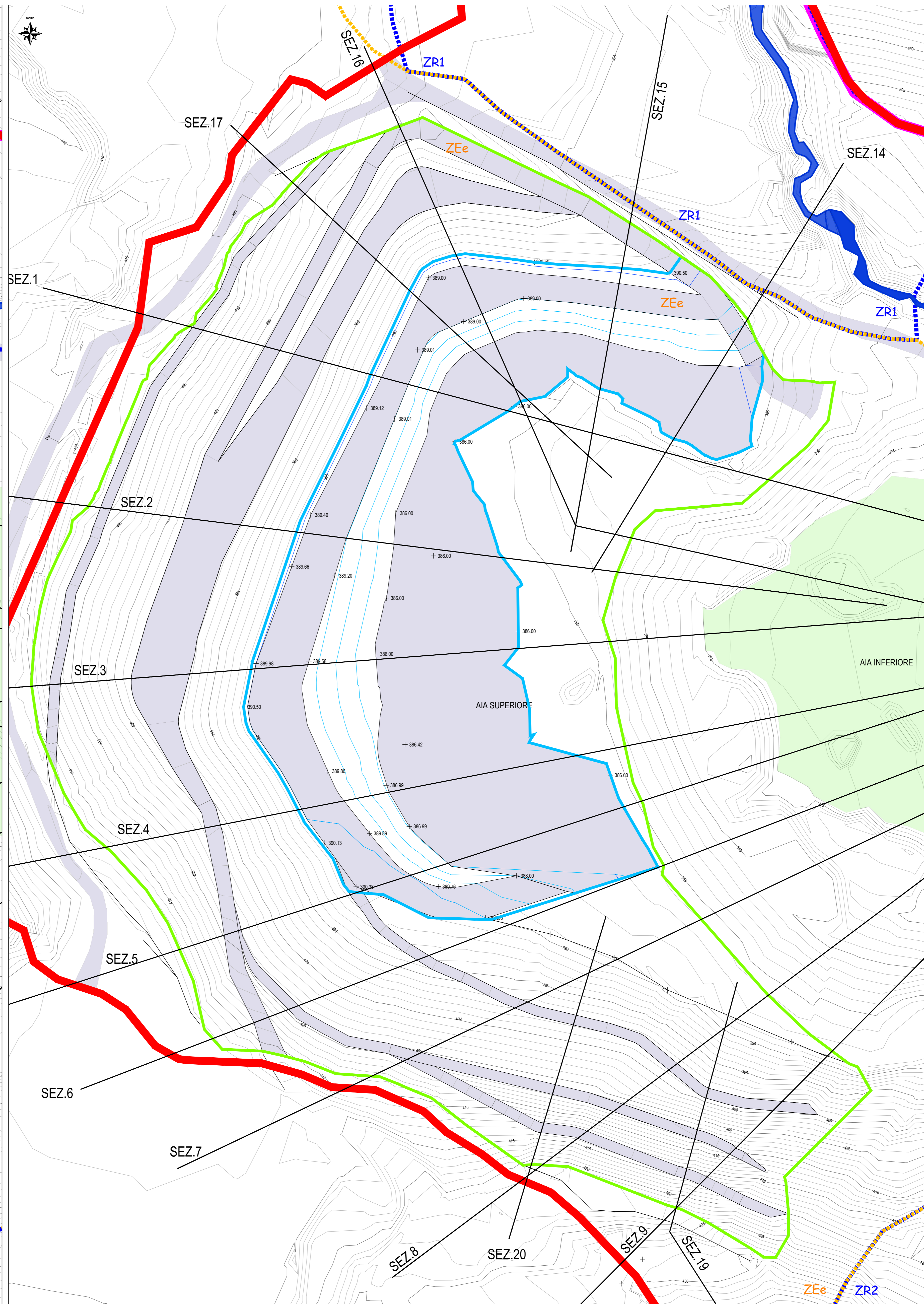
PLANIMETRIA DI PROGETTO DI COLTIVAZIONE - ANNO 4 - SCALA 1:750
